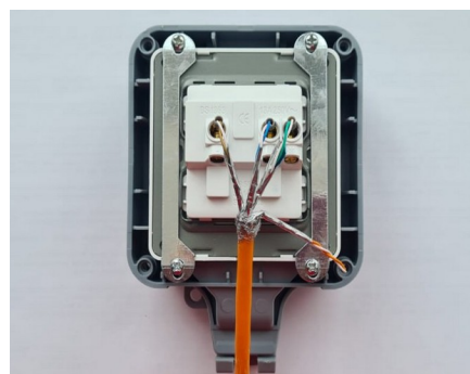
S/FTP cable
